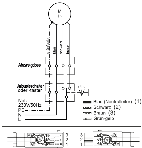
Fig. 4 Schaltbild RolTop L RH 230 V / 50 Hz und Kabelbelegung bei Verwendung mit Hirschmann-Steckverbindung STAS-3
