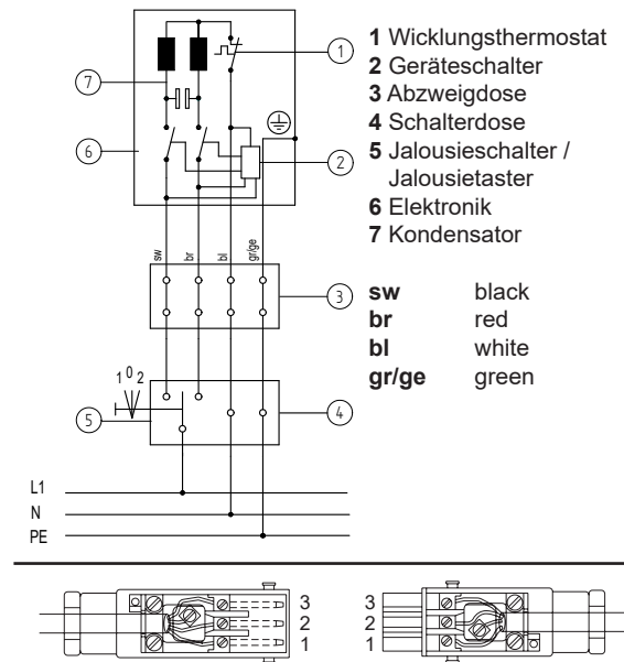
Fig. 5 Schaltbild SunTop/Z M RH 120 V / 60 Hz und Kabelbelegung bei Verwendung mit Hirschmann-Steckverbindung STAS-3
