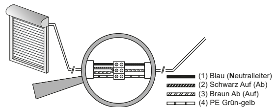
Fig. 7 Anschluss Funksendebetrieb
