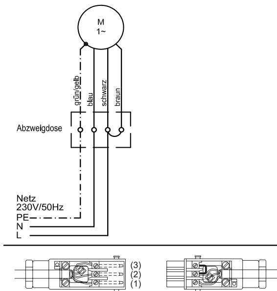
Fig. 5 Schaltbild RolMotion/D+ M-868 230V / 50Hz und Kabelbelegung bei Verwendung mit Hirschmann-Steckverbindung STAS-3 (mit Brücke)
